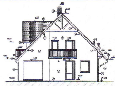
POHLED ZADNÍ
