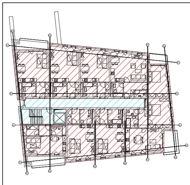
Obr. 3 – půdorys 3NP
