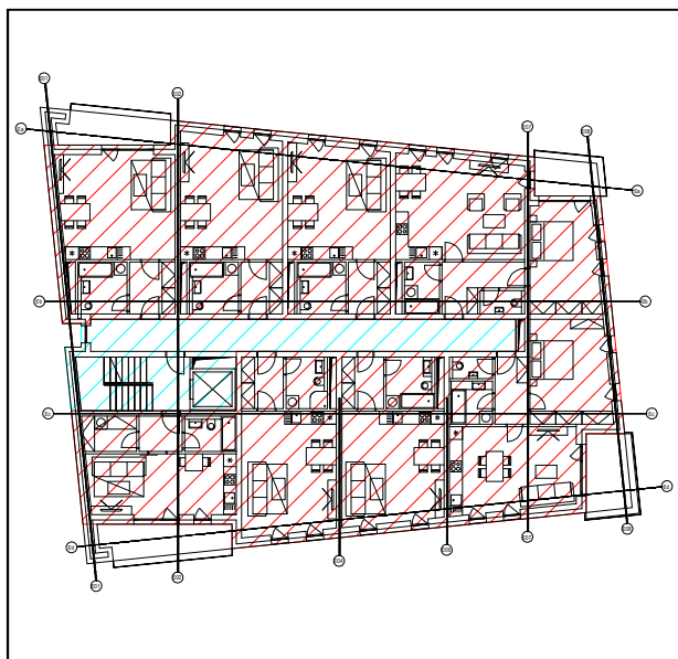
Obr. 4 – půdorys 4NP
