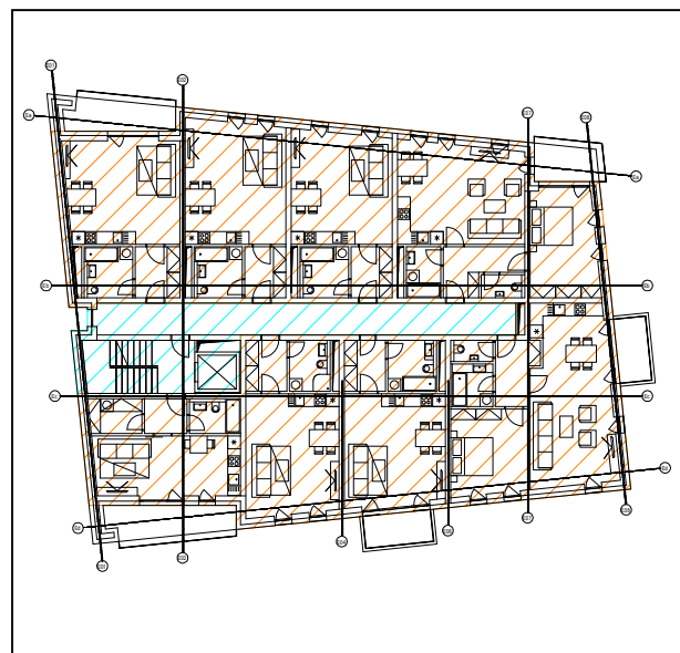
Obr. 4 – půdorys 4NP
