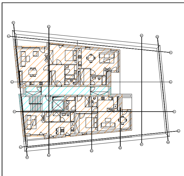
Obr. 7 – půdorys 7NP
