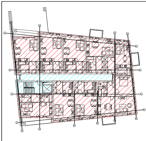
Obr. 2 – půdorys 2NP
