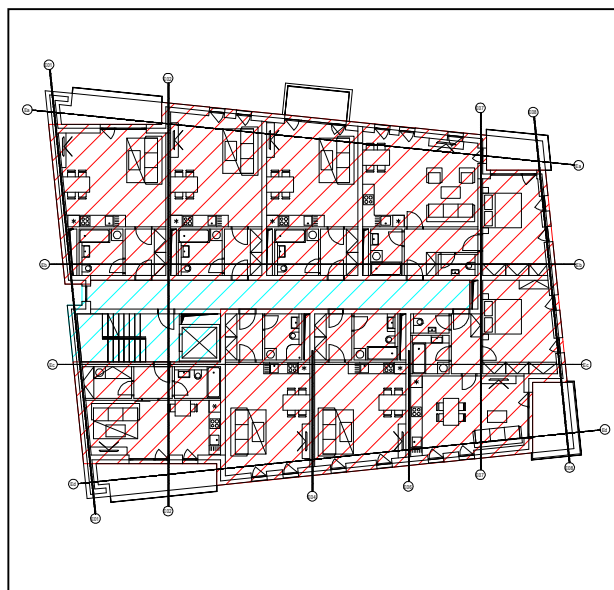
Obr. 3 – půdorys 3NP
